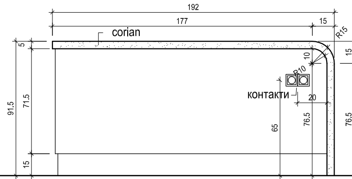
Изглед 5 М 1:25
