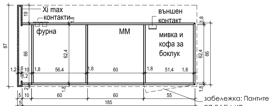
Разрез 1 М 1:25
