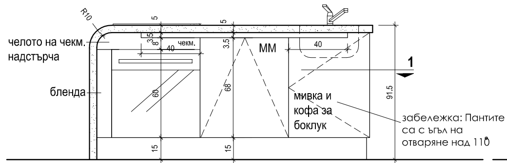
Изглед 4 М 1:25
