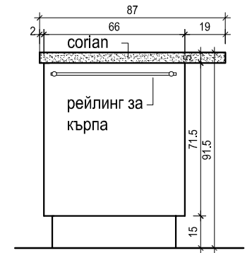
Изглед 3 М 1:25
