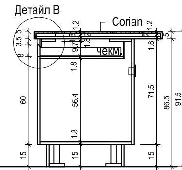
Разрез 2 М 1:25
