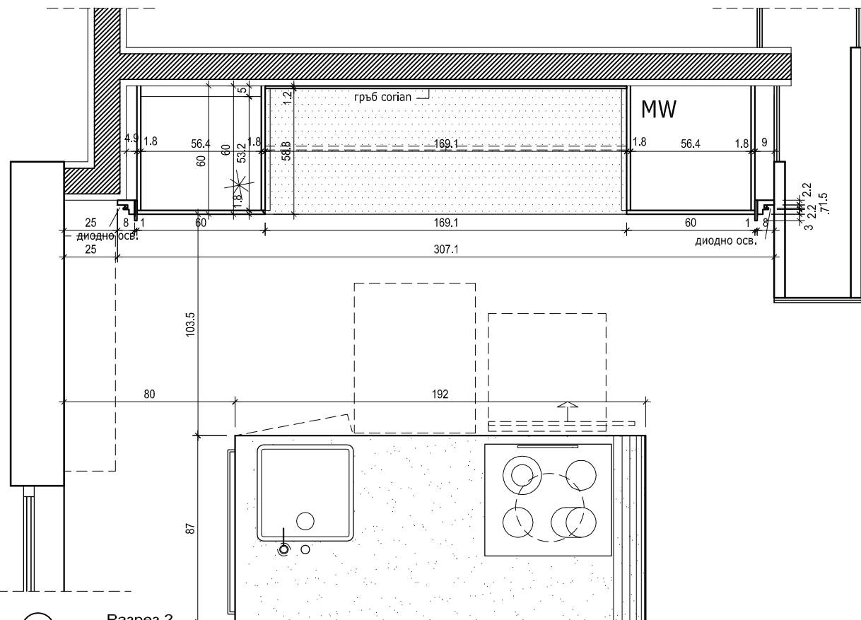
1 Разрез 2 М 1:25
