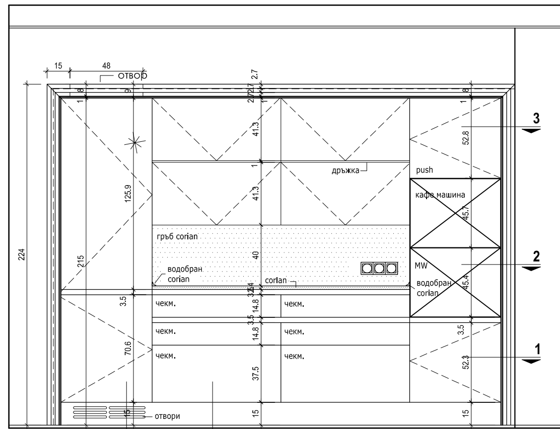
1 Изглед М 1:25
