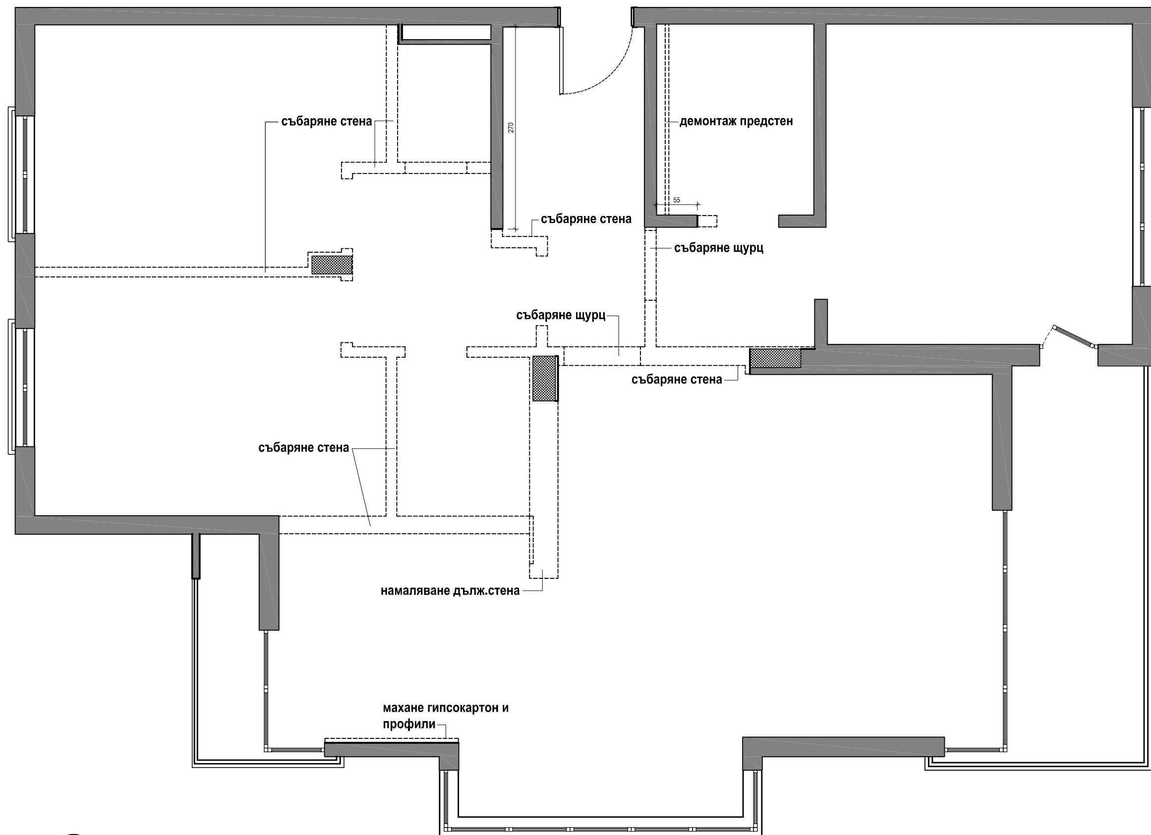
1 ПЛАН СЪБАРЯНЕ М 1:50
